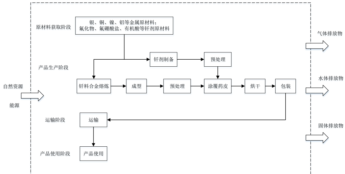
图 B.1 药皮钎料生命周期系统边界图
