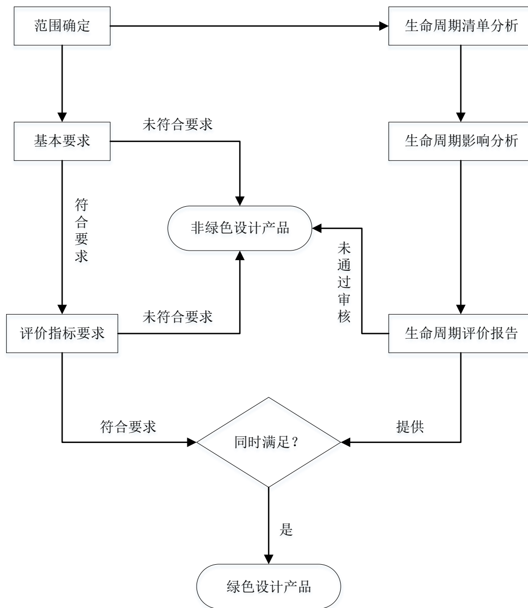
图 1 药皮钎料绿色设计产品评价流程
